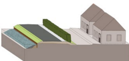
I 4a: Ophoging rijbaan i.c.m. bodemverzwaring
